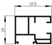
Geleider heroal VS Z
