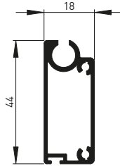
heroal VS Z Onderlijst Type II
