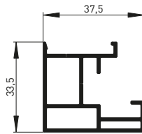
Geleider heroal VS Z Contra
