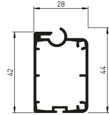
heroal VS Z Onderlijst Type III
