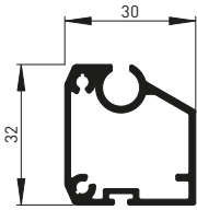
heroal VS Z Onderlijst Type I
