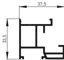
Geleider tweedelig
